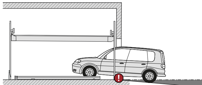
max. 5% gradient
